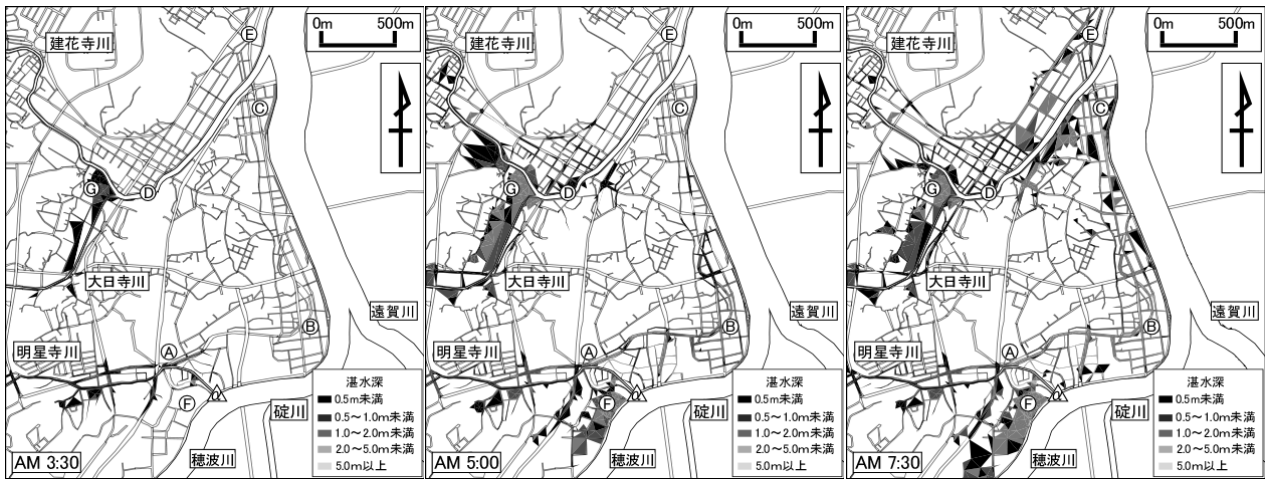
図-10 氾濫プロセス (AM3:30 (左), AM5:00 (中), AM7:30 (右))
