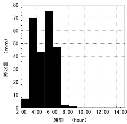
図-6 解析に用いたハイトグラフ
