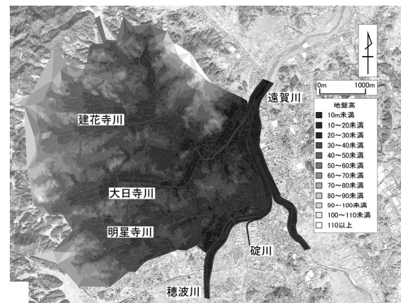
図-4 解析データ（地盤高コンター）
