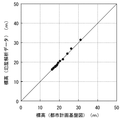
図-5 標高の比較
