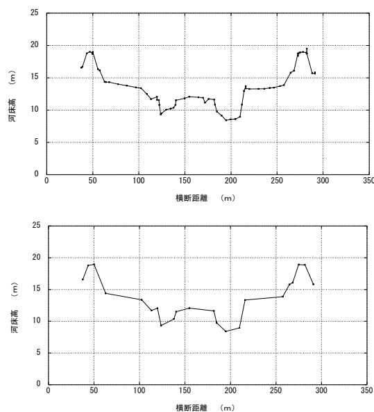
図-2 横断面図(上)と線形補完した(下)横断面図
