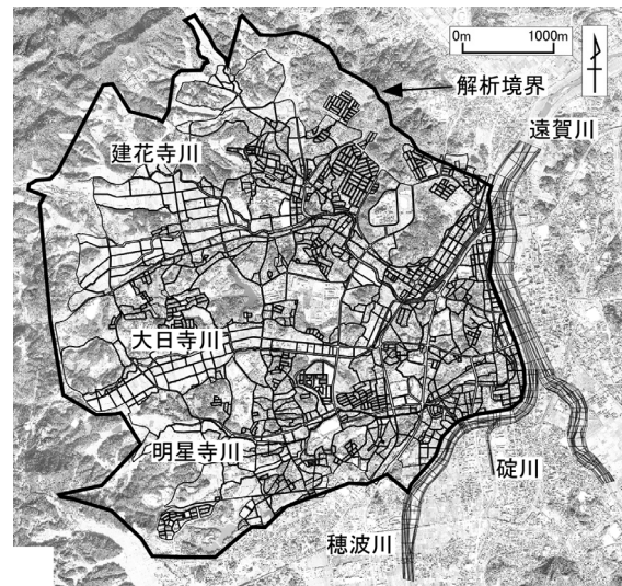
図-3 街区と河道の堤防・低水路線形
