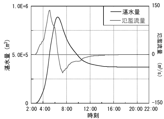
図-11 湛水量・氾濫流量の経時変化
