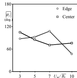
図-8 降下魚が潜孔下流領域へ進入したときの魚向 ( U_m : 潜孔内流速, B_L : カワムツの平均体長, |\theta_f| : 魚向 \theta_f の絶対値の平均値)
