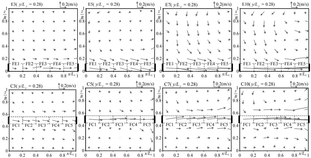
図2 第2プール内の水平面内流速ベクトル ( B :魚道幅, L_x :プール長, L_y :水深, FE1~FE5, FC1~FC5:潜孔下流領域を5等分した領域)
