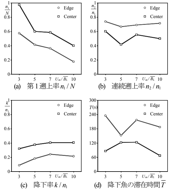
図-4 潜孔内流速の変化による第1遡上率 n_1/N , 連続遡上率 n_2/n_1 , 降下率 k/n_1 および, 降下魚の滞在時間 \bar{T} の変化 ( B :魚道幅, L_x :プール長, L_y :水深, N :実験に用いたカワムツの尾数, U_m :潜孔内流速, \bar{B}_L :カワムツの平均体長)
