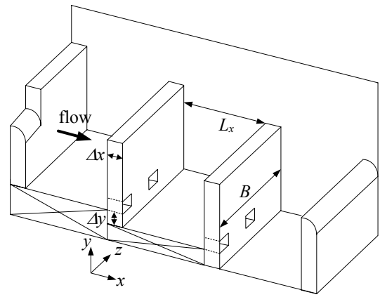
図-1 実験に用いた魚道の概要
